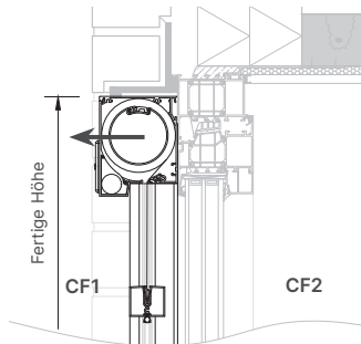
Vorbau, vor dem Fenster, mit vollständig verarbeiteter Kassette
